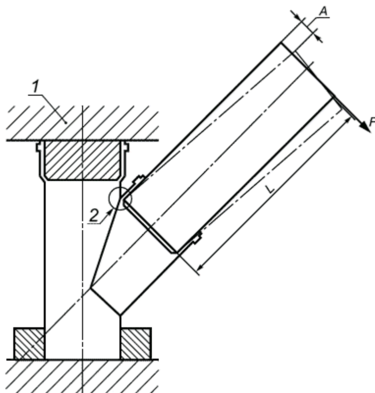
1 - фиксирующие элементы; 2 - зона возможного разрушения
