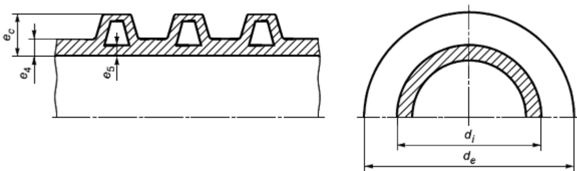
е) Тип В (с кольцевым полым профилем)
