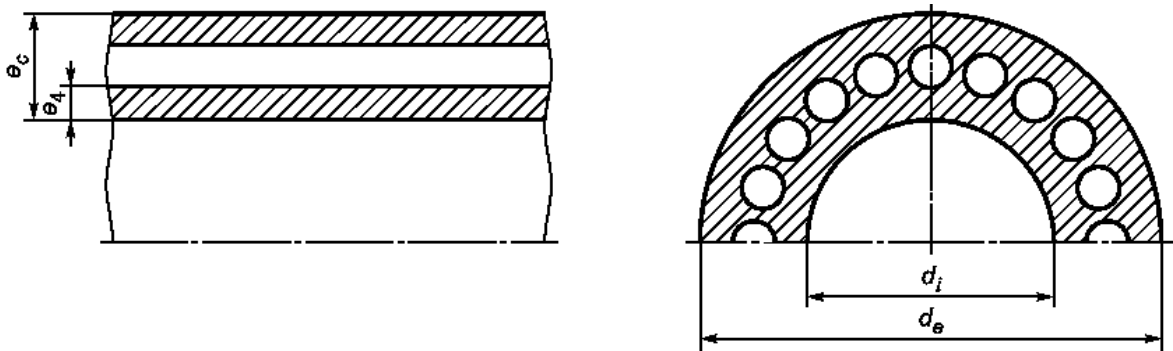
б) Тип А1 (с продольными полыми секциями)
