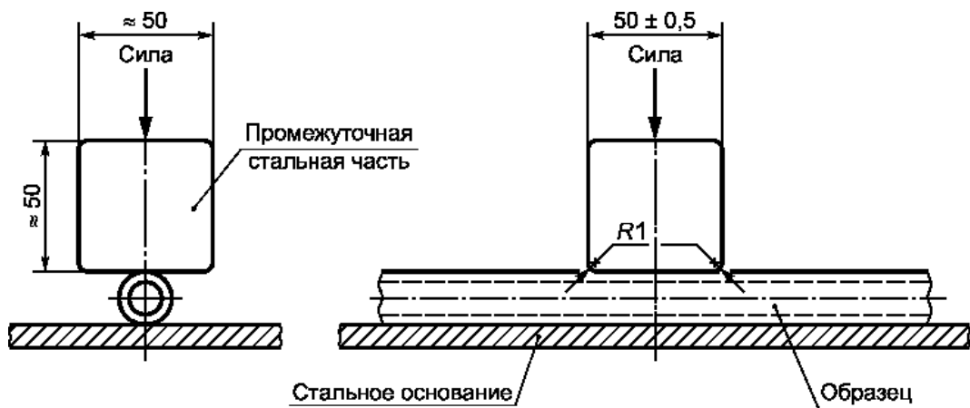
Рисунок 1 - Установка для испытаний на сжатие
