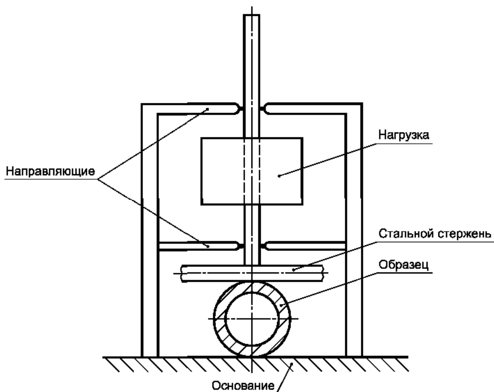
Рисунок 8 - Стенд испытаний на сопротивление высокой температуре
